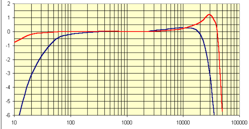
Eintakt-AÜ 53.05, EL84 mit 1/2 6N3P als Vorstufe, blau ohne GK , rot mit GK 5K / 390R in die Vorstufenkathode
