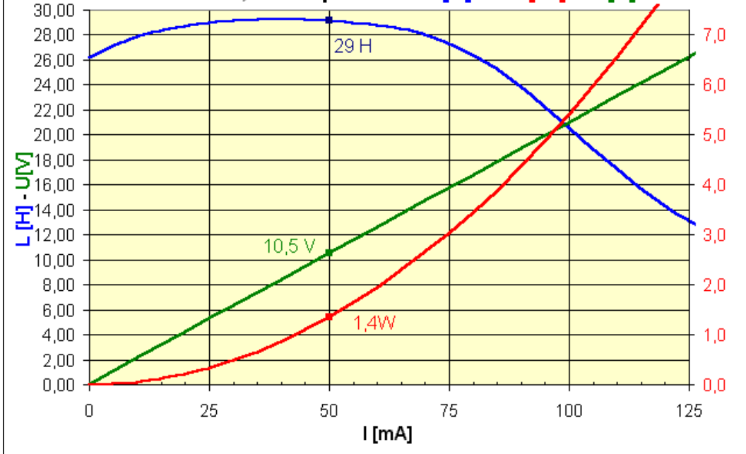
AÜ 53.05, 1Veff primär L[H] - Pv[W] - U[V]
